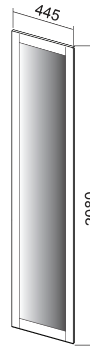
Дверь с зеркалом ПМ-241.07.01.000 ТД 241.07.12
