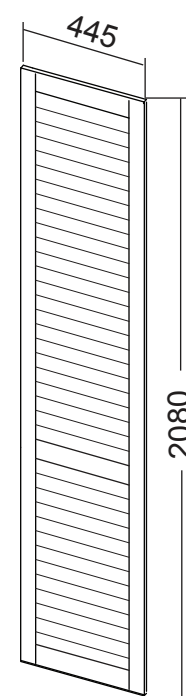
Дверь правая/левая ПМ-241.21.01.000 ТД 241.07.11R/L
